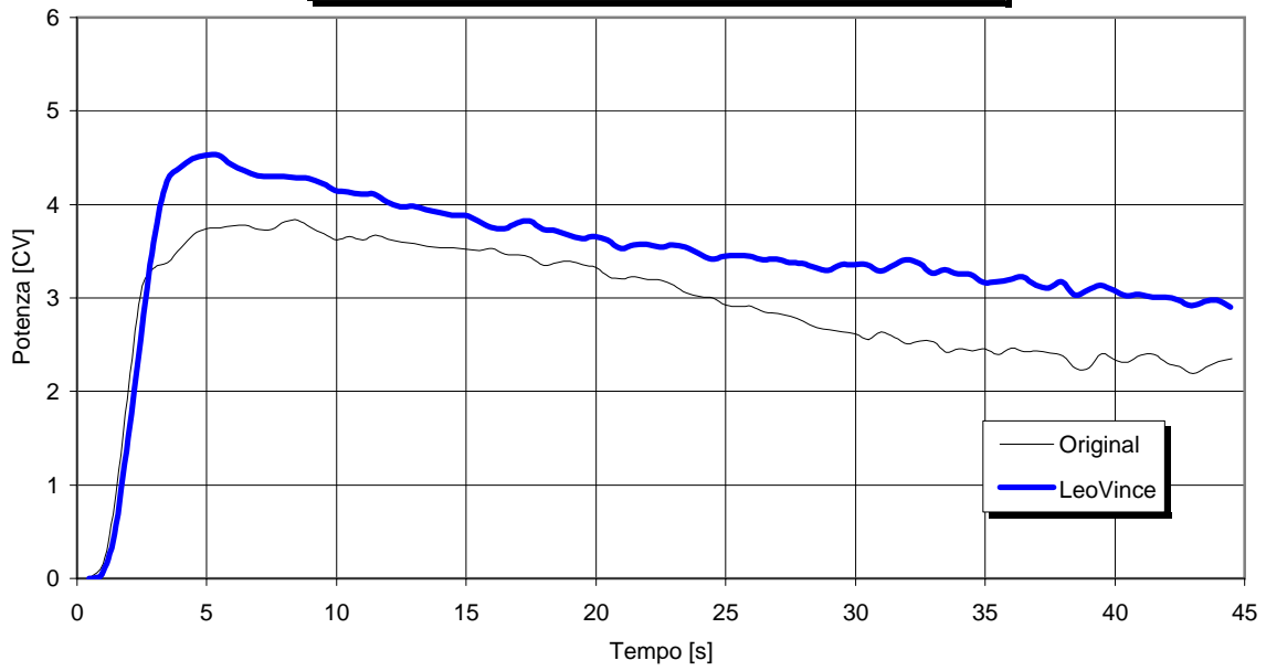
APRILIA SR 50 R FACTORY ('04/'07 - carburatori)
