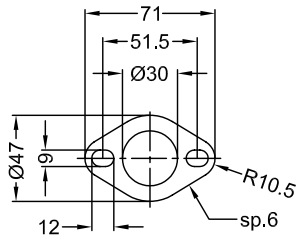
Vista da "B" Flangia "43D"
