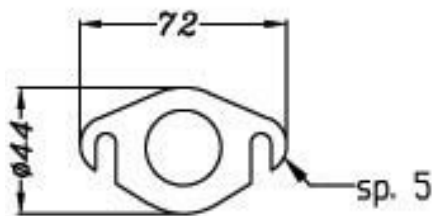
Vista da "A" Flangia "99A"
