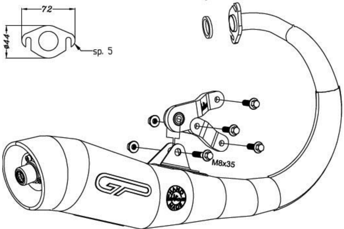
Vista da "A" Flangia "99A"
